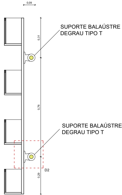
VISTA LATERAL COM FIXADOR ESCALA: 1/100
