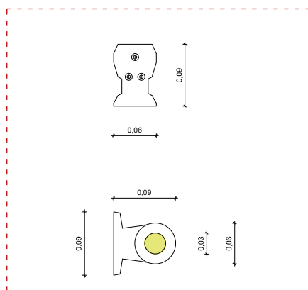
SUPORE BALAUÍSTRE DEGRAU TIPO T ESCALA: 1/5
