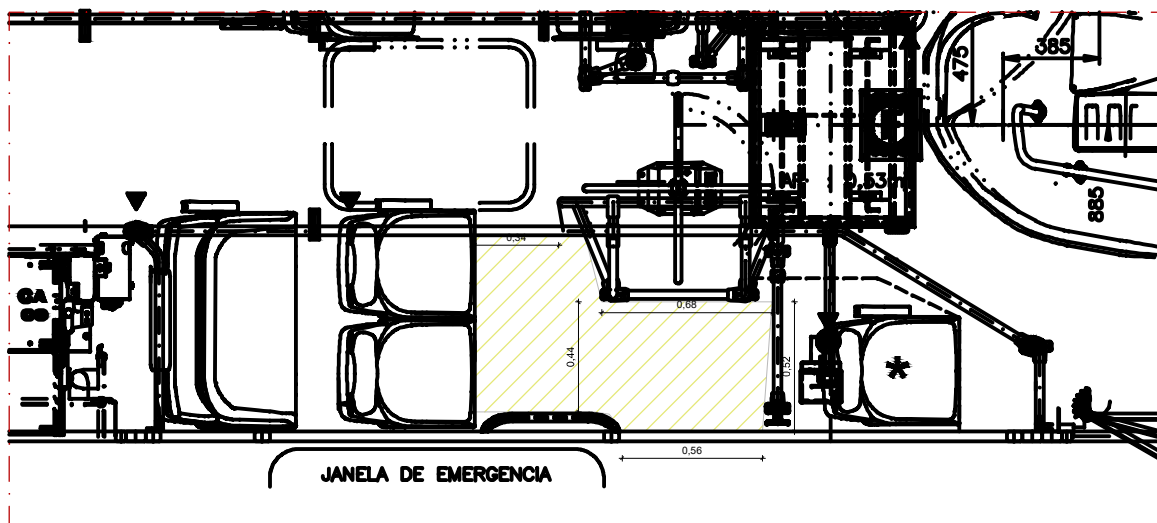
ÁREA PREVISTA PARA IMPLANTAÇÃO (Marcopolo Torino 5 Portas 2019 - ROD) ESCALA: 1/200
