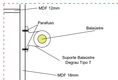
DETALHAMENTO D2 (FIXAÇÃO) ESCALA: 1/5
