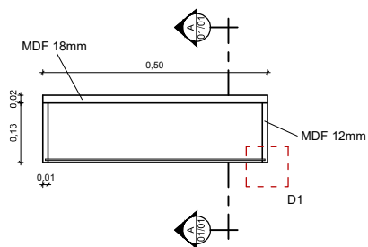
PLANTA BAIXA ESCALA: 1/100
