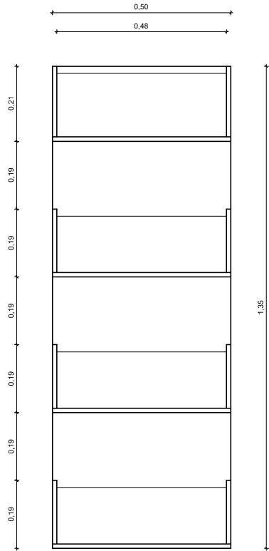
VISTA FRONTAL DA ESTRUTURA ESCALA: 1/100
