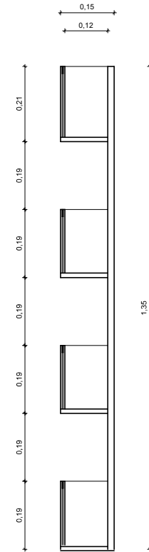
CORTE AA' ESCALA: 1/100
