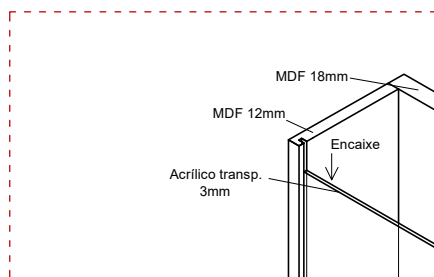
DETALHAMENTO D1 (PERSPECTIVA) ESCALA: 1/5
